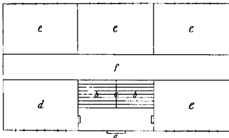
Grundriß des Erdgeschosses eines Schulgebäudes. Maßstab 1:300. a Eingang, b Treppenausgang, c Geländer, d Wohnung des Direktors, e Lehrstühle, f Gang.
